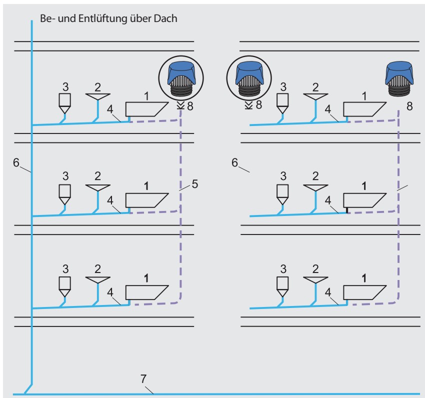
Belüftung von Falleleitungen mit ventilair®
